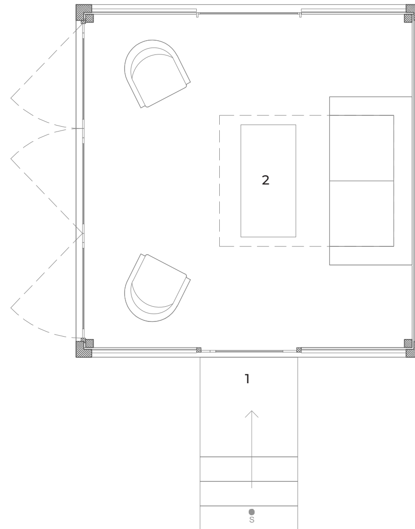
PLANTA BAJA
