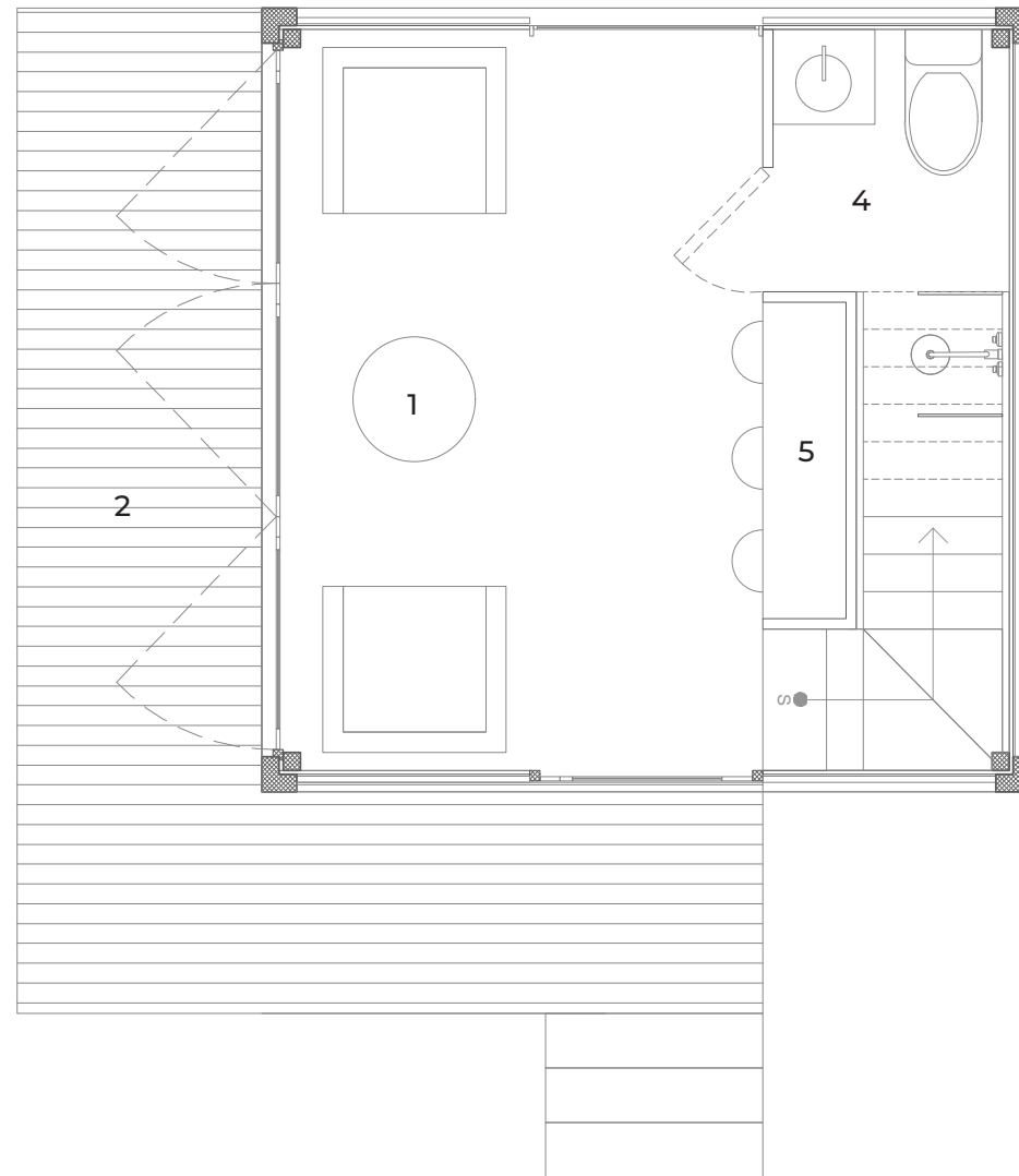
PLANTA BAJA
